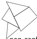
non conforming
